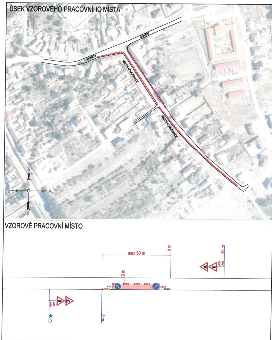
Obrázek 1 – situace dopravního značení
